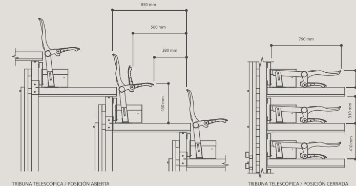
TRIBUNA TELESCÓPICA / POSICIÓN ABIERTA
